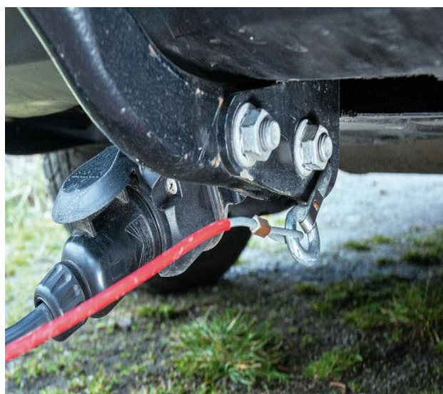
Ilustracja nr 2- sposób zaczepienia linki awaryjnej-hak demontowany
